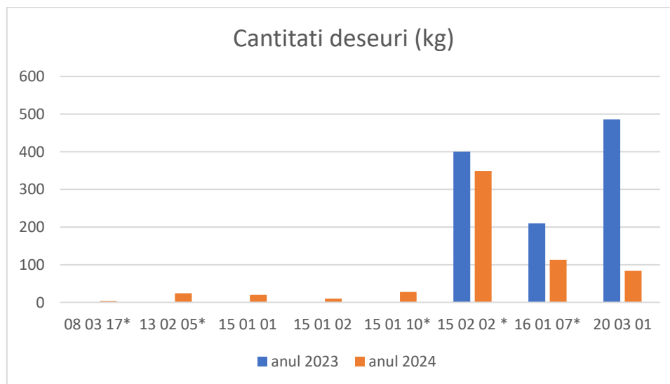
Figura 1: Cantitate (kg) anuală de deșeuri generată la nivelul anilor 2023 și 2024 – CEE Ciocârlia-Cobadin
